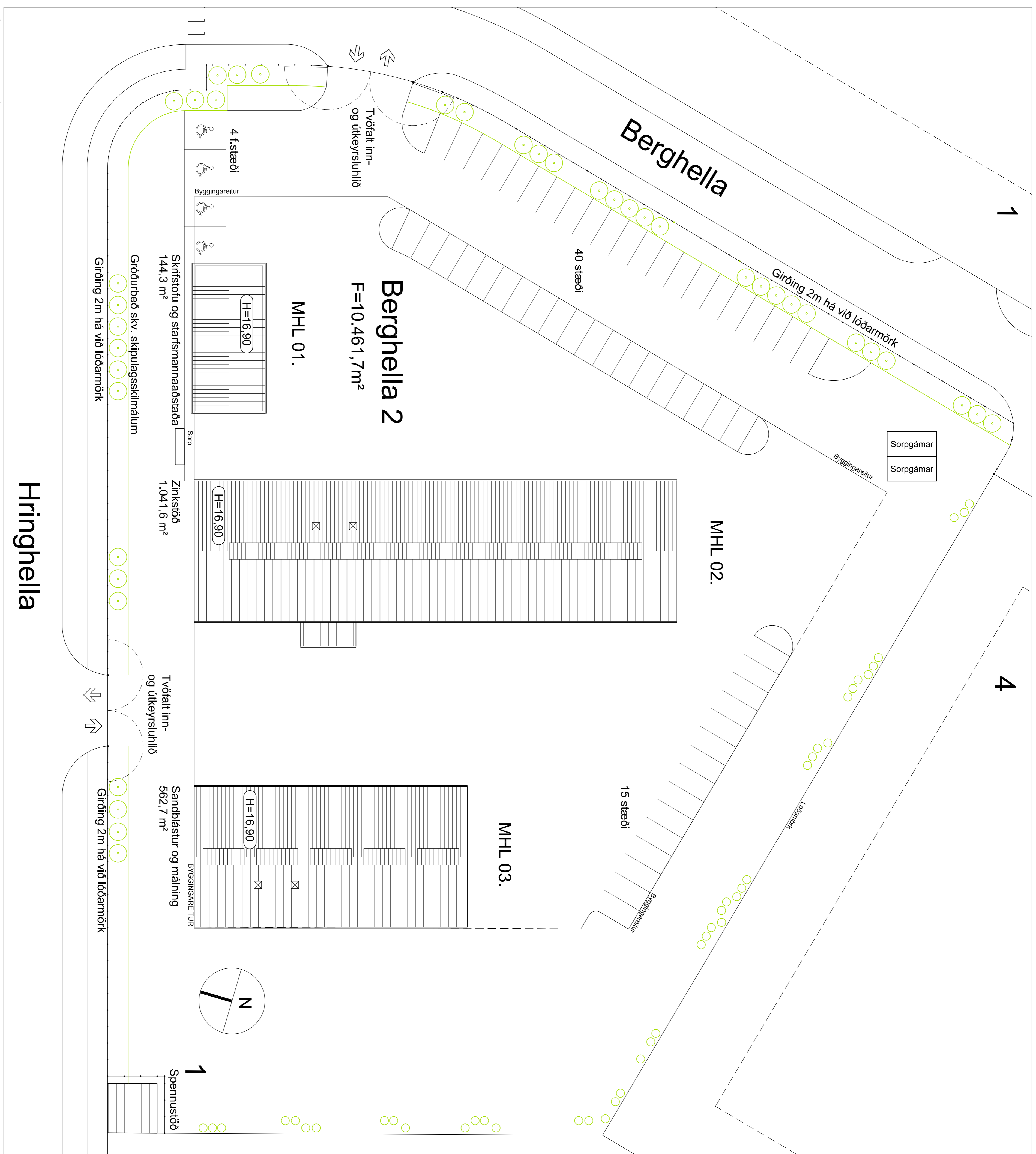
LÓÐARUPPDRATTUR 1:250
